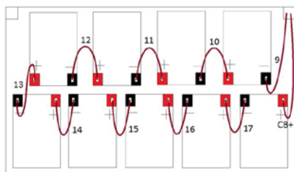
Övre hylla (ovanifrån)
