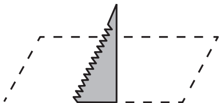
Edge S, urtagningshål (vägg/tak) 310x310 mm
